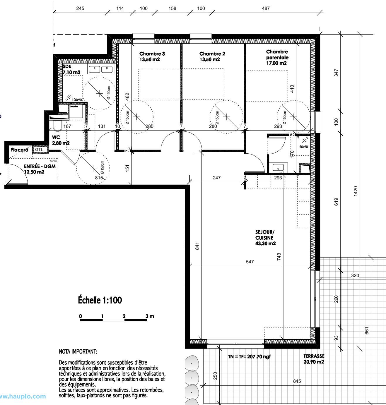
PLAN RDC
